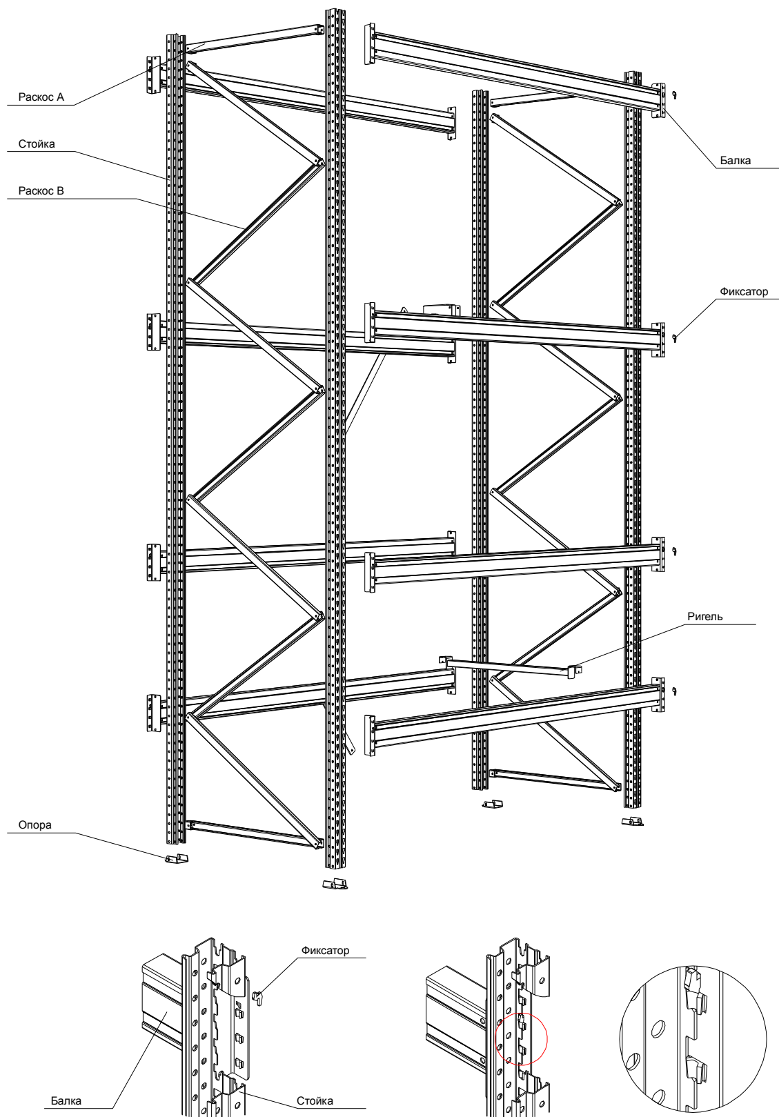
Схема сборки фронтального складского стеллажа
