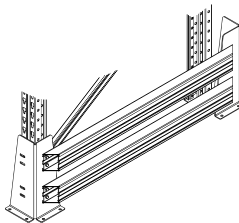
Боковой отбойник
